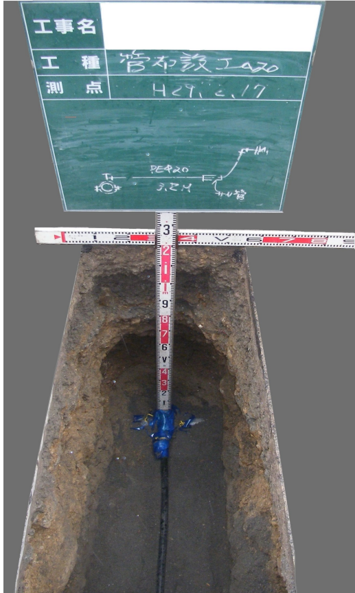
分岐道路内配管施工状況
