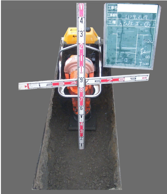
埋戻し完了状況
